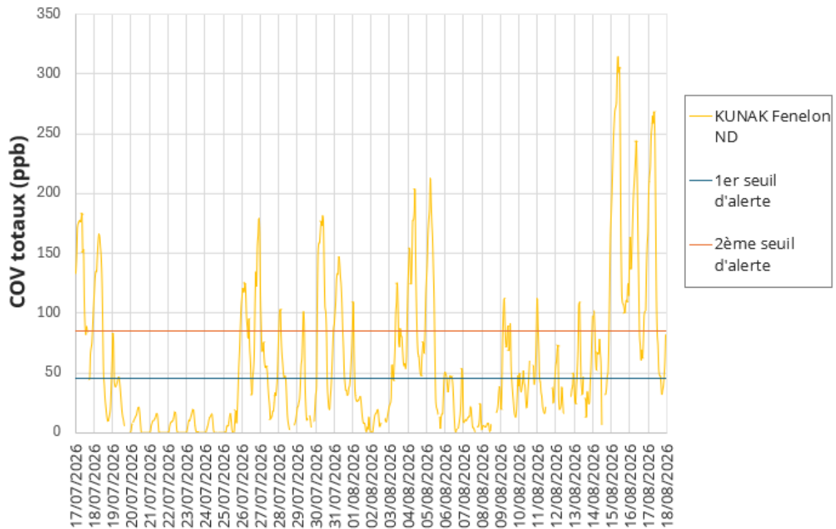
Figure 12 : Evolution des concentrations moyennes horaires en COV totaux au point de mesure, du 17 juillet au 17 août 2026 inclus
