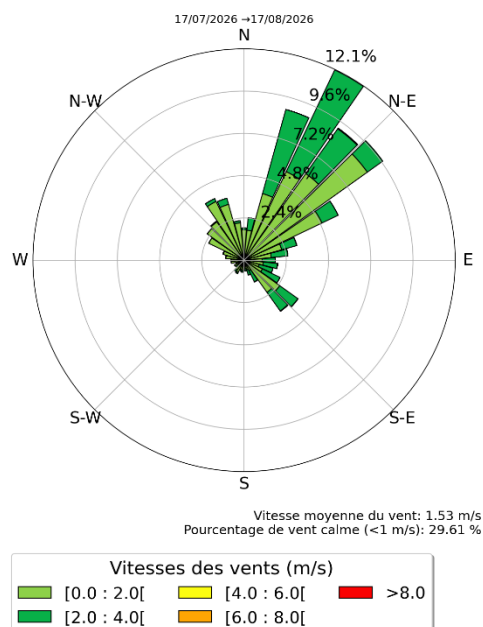
Figure 8 : Rose des vents Fénélon ND du 17 juillet au 17 août 2026 inclus – données issues du capteur KUNAK
