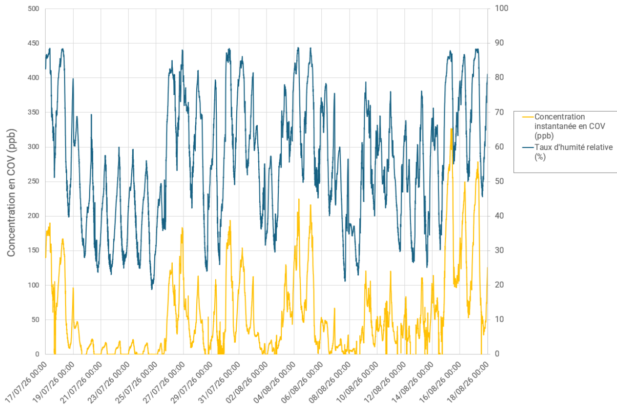
Figure 13 : Evolution des concentrations instantanées en COV totaux et du taux d'humidité relative au point de mesure, du 17 juillet au 17 août 2026 inclus
