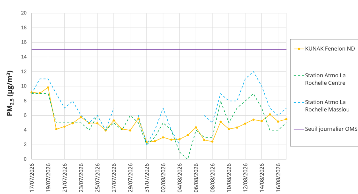
Figure 11 : Evolution des concentrations moyennes journalières en PM_{2,5} au point de mesure et aux stations d'Atmo Nouvelle-Aquitaine retenues, du 17 juillet au 17 août 2026 inclus
