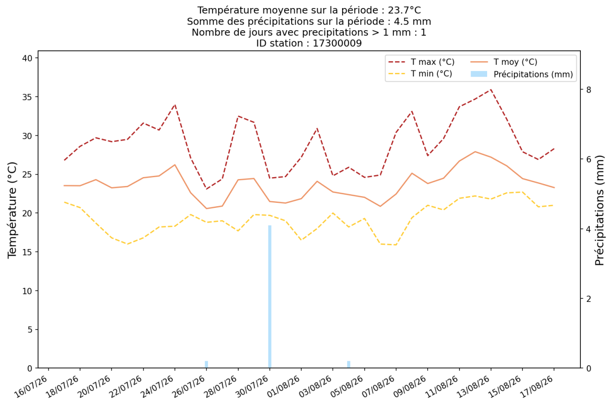
Figure 6 : Températures et précipitations du 17 juillet au 17 août 2026 inclus à la station La Rochelle – Ile-de-Ré
