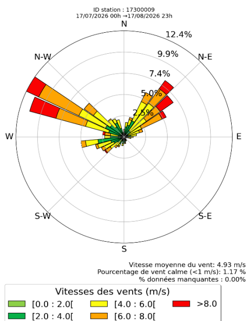
Figure 7 : Rose des vents à la station La Rochelle – Ile-de-Ré du 17 juillet au 17 août 2026 inclus – données issues de Météo France
