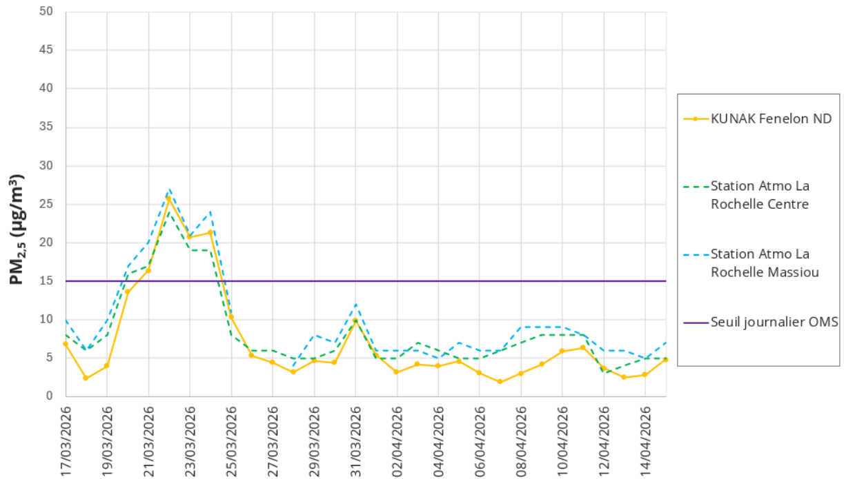
Figure 10 : Evolution des concentrations moyennes journalières en \text{PM}_{2,5} au point de mesure et aux stations d'Atmo Nouvelle-Aquitaine retenues, du 17 mars au 15 avril 2026 inclus
