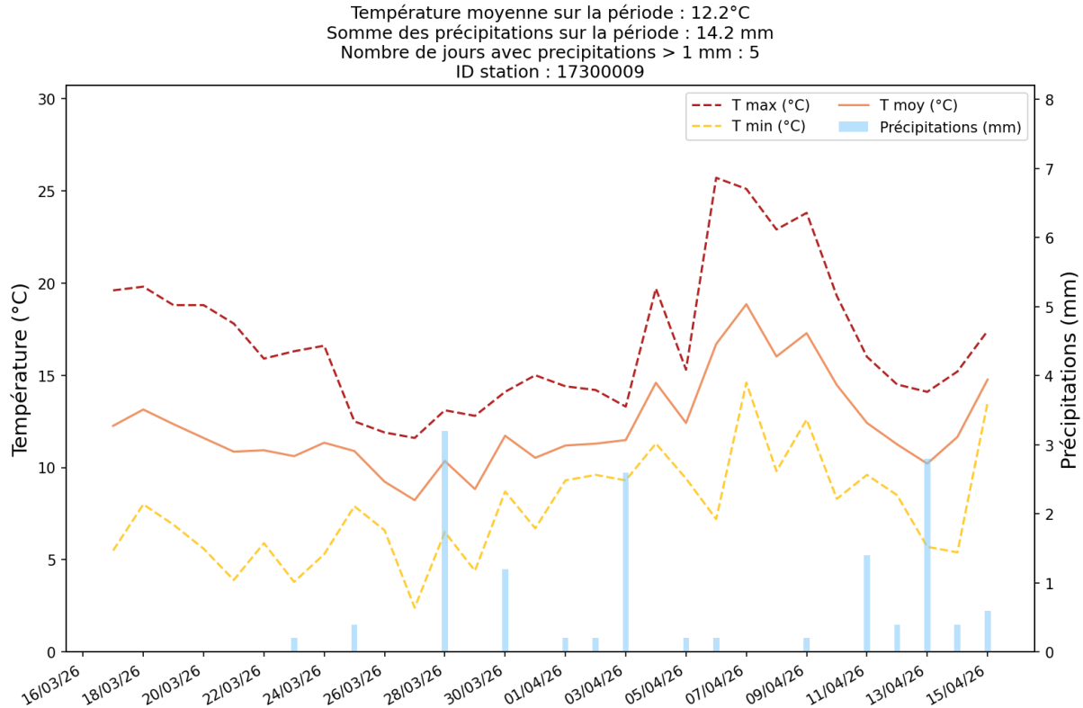
Figure 5 : Températures et précipitations du 17 mars au 15 avril 2026 inclus à la station La Rochelle – Ile-de-Ré
