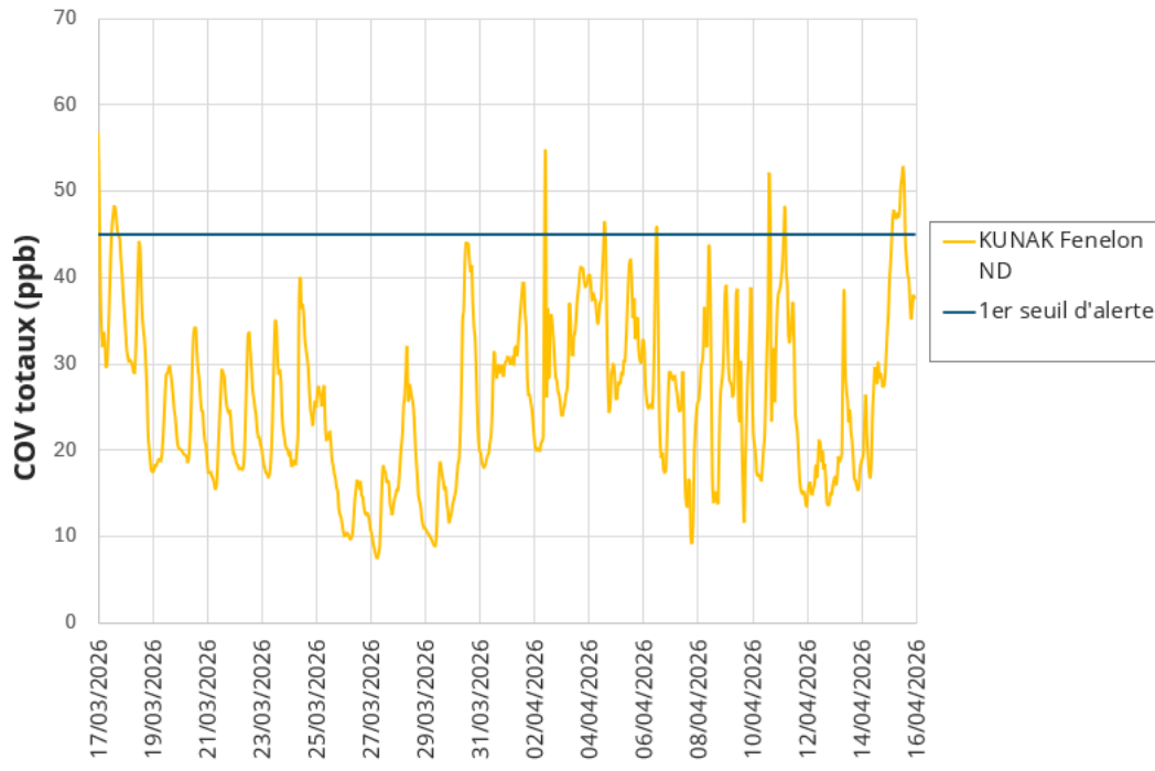
Figure 11 : Evolution des concentrations moyennes horaires en COV totaux au point de mesure, du 17 mars au 15 avril 2026 inclus
