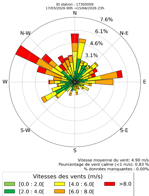
Figure 6 : Rose des vents à la station La Rochelle – Ile-de-Ré du 17 mars au 15 avril 2026 inclus – données issues de Météo France
