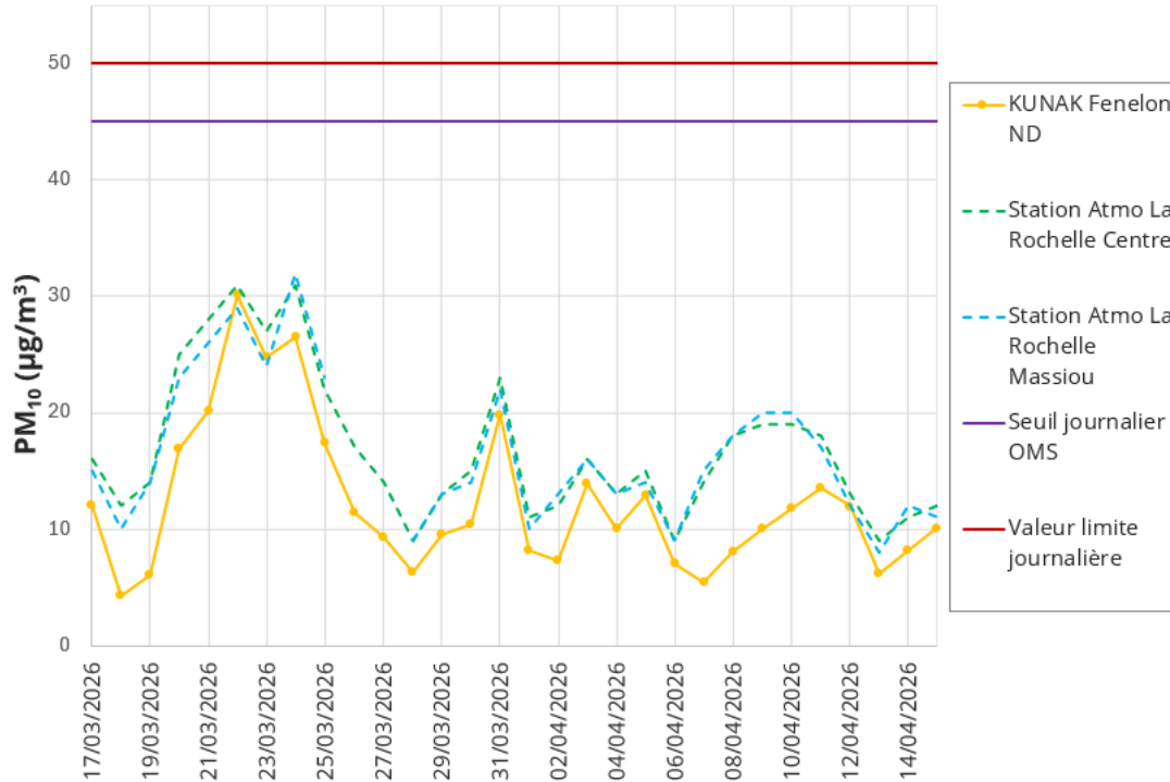
Figure 9 : Evolution des concentrations moyennes journalières en PM 10 au point de mesure et aux stations d'Atmo Nouvelle-Aquitaine retenues, du 17 mars au 15 avril 2026 inclus
