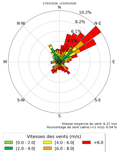
Figure 7 : Rose des vents Fénelon ND du 17 mars au 15 avril 2026 inclus – données issues du capteur KUNAK
