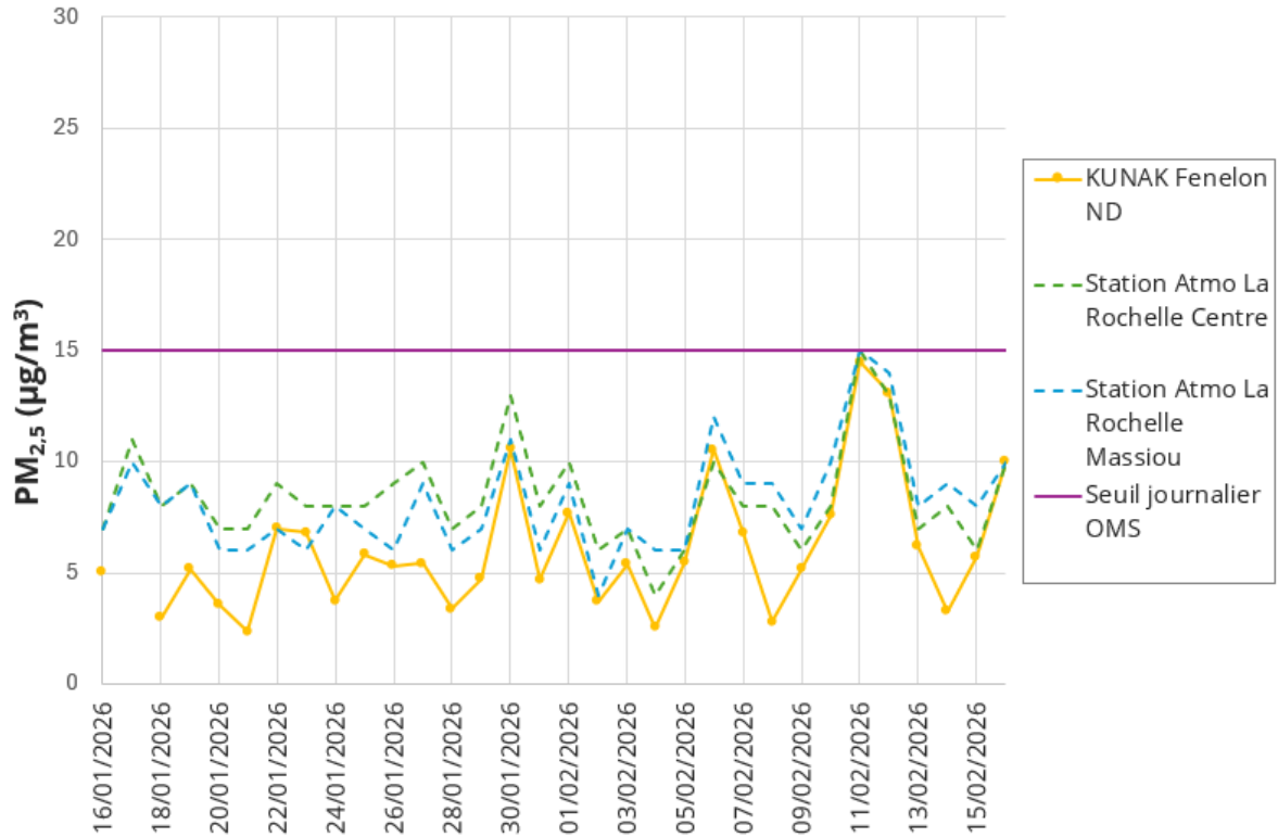
Figure 10 : Evolution des concentrations moyennes journalières en \text{PM}_{2,5} au point de mesure et aux stations d'Atmo Nouvelle-Aquitaine retenues, du 16 janvier au 16 février 2026 inclus
