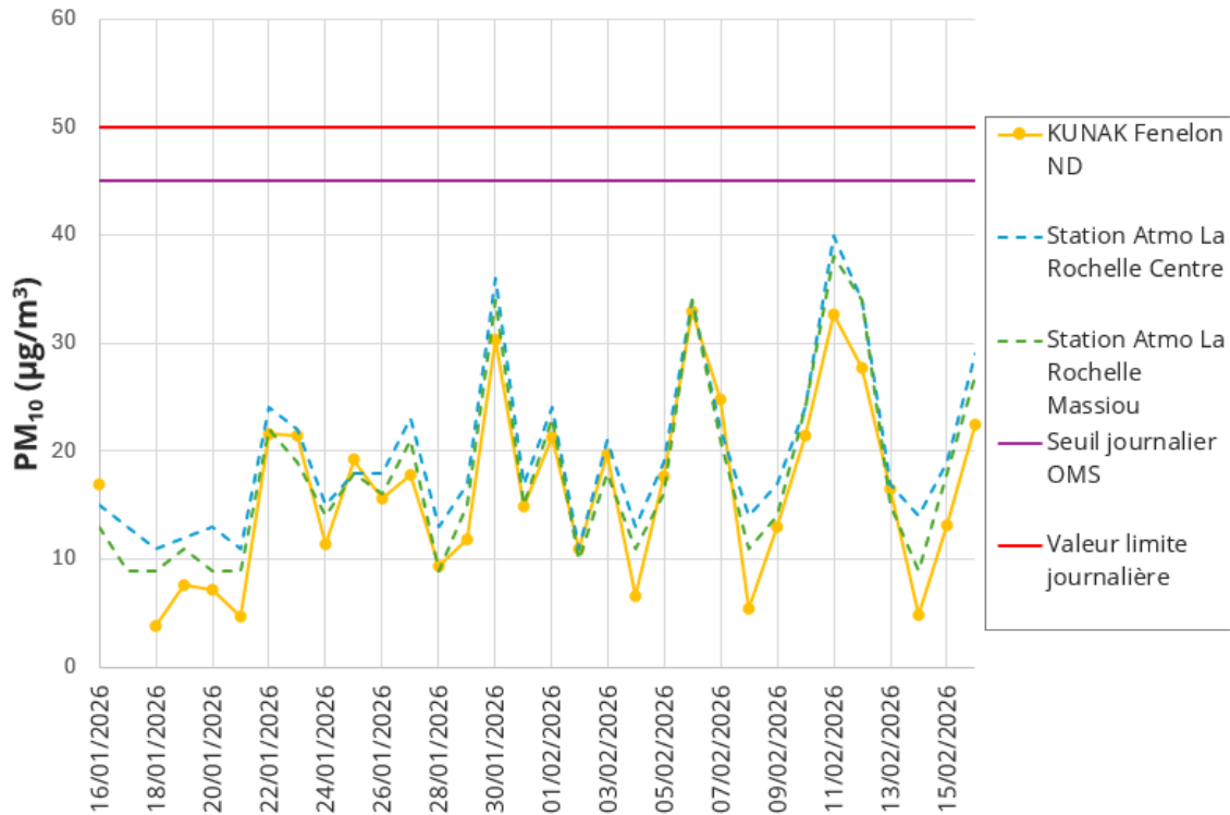
Figure 9 : Evolution des concentrations moyennes journalières en PM 10 au point de mesure et aux stations d'Atmo Nouvelle-Aquitaine retenues, du 16 janvier au 16 février 2026 inclus
