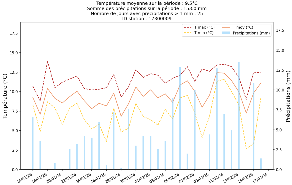
Figure 5 : Températures et précipitations du 16 janvier au 16 février 2026 inclus à la station La Rochelle – Ile-de-Ré
