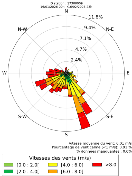
Figure 6 : Rose des vents à la station La Rochelle – Ile-de-Ré du 16 janvier au 16 février 2026 inclus – données issues de Météo France
