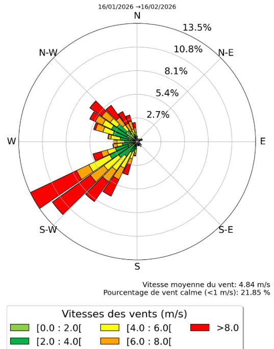
Figure 7 : Rose des vents Fénelon ND du 16 janvier au 16 février 2026 inclus – données issues du capteur KUNAK
