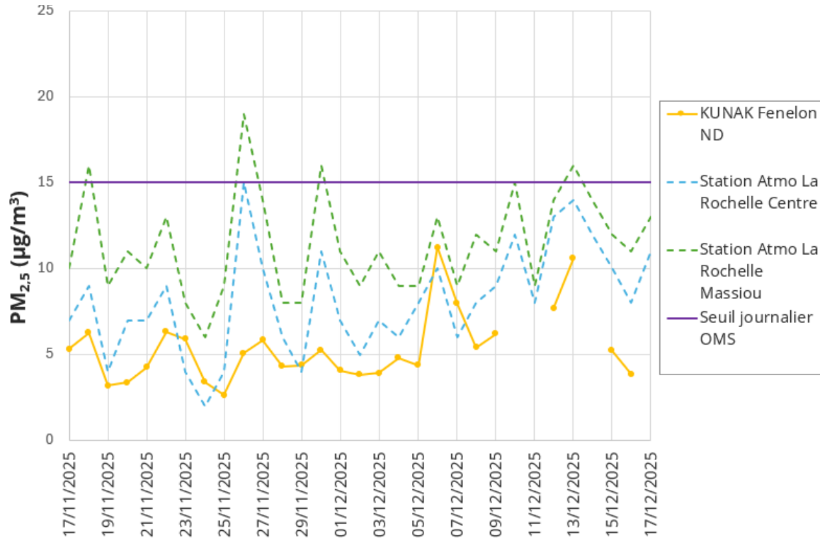
Figure 10 : Evolution des concentrations moyennes journalières en PM 2,5 au point de mesure et aux stations d'Atmo Nouvelle-Aquitaine retenues, du 17 novembre au 17 décembre 2025 inclus
