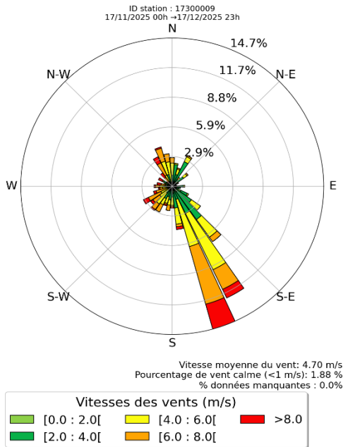
Figure 6 : Rose des vents à la station La Rochelle – Ile-de-Ré du 17 novembre au 17 décembre 2025 inclus – données issues de Météo France
