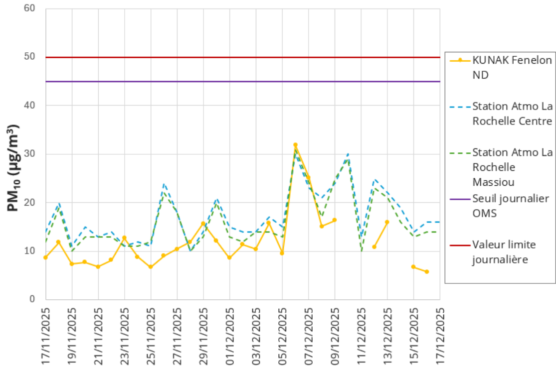
Figure 9 : Evolution des concentrations moyennes journalières en PM 10 au point de mesure et aux stations d'Atmo Nouvelle-Aquitaine retenues, du 17 novembre au 17 décembre 2025 inclus
