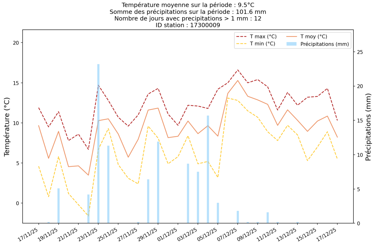
Figure 5 : Températures et précipitations du 17 novembre au 17 décembre 2025 inclus à la station La Rochelle – Ile-de-Ré
