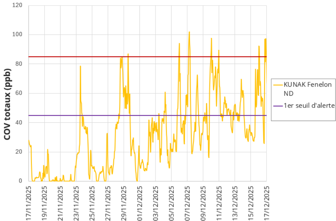
Figure 11 : Evolution des concentrations moyennes horaires en COV totaux au point de mesure, du 17 novembre au 17 décembre 2025 inclus
