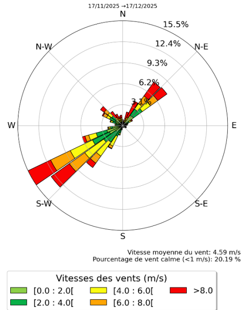
Figure 7 : Rose des vents Fénelon ND du 17 novembre au 17 décembre 2025 inclus – données issues du capteur KUNAK
