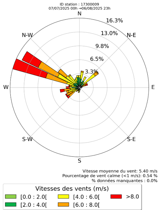
Figure 6 : Rose des vents à la station La Rochelle – Ile-de-Ré du 7 juillet au 6 août 2025 – données issues de Météo France
