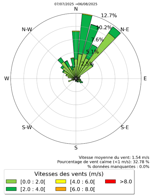
Figure 7 : Rose des vents Fénelon ND du 7 juillet au 6 août 2025 – données issues du capteur KUNAK
