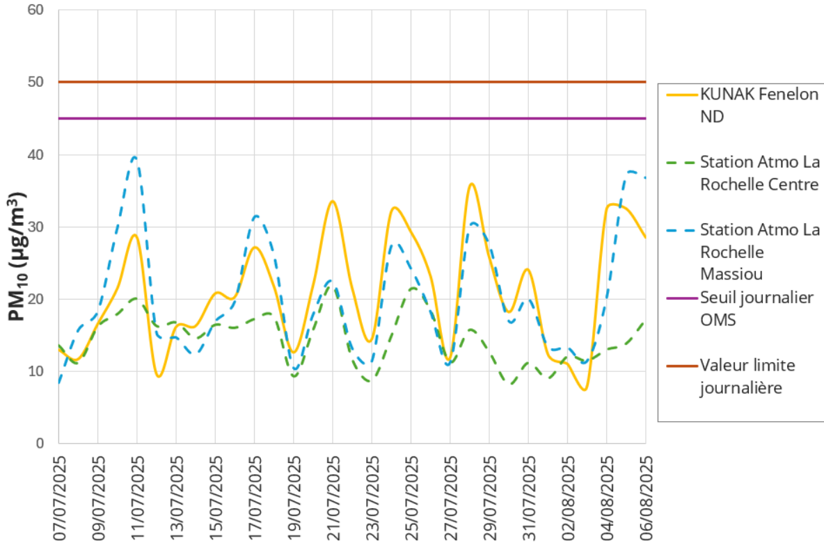
Figure 9 : Evolution des concentrations moyennes journalières en PM 10 au point de mesure et aux stations d'Atmo Nouvelle-Aquitaine retenues, du 7 juillet au 6 août 2025
