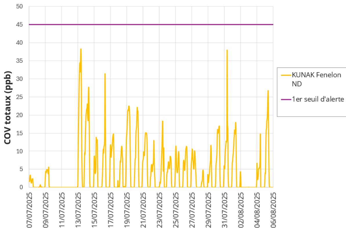
Figure 11 : Evolution des concentrations moyennes horaires en COV totaux au point de mesure, du 7 juillet au 6 août 2025
