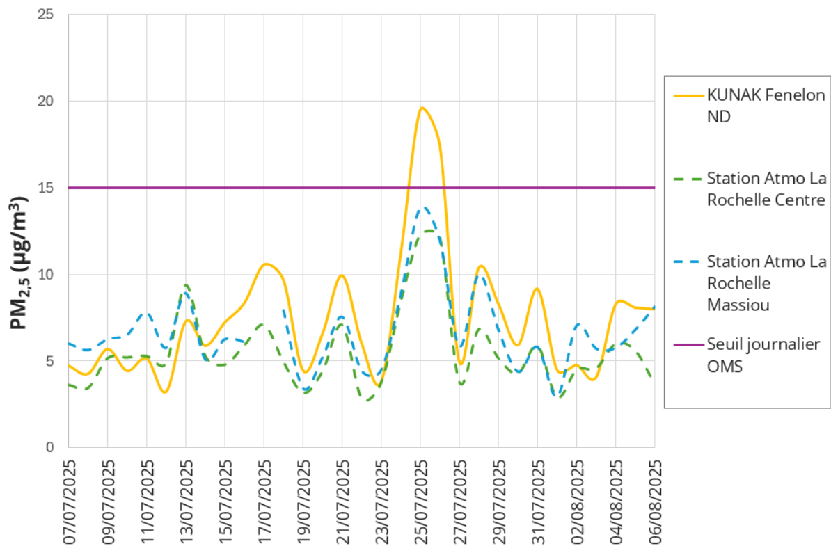
Figure 10 : Evolution des concentrations moyennes journalières en \text{PM}_{2,5} au point de mesure et aux stations d'Atmo Nouvelle-Aquitaine retenues, du 7 juillet au 6 août 2025
