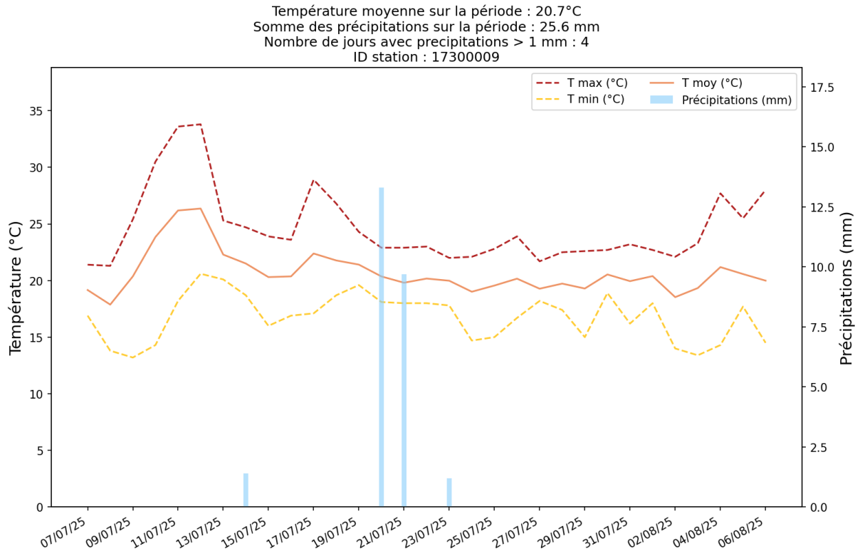
Figure 5 : Températures et précipitations du 7 juillet au 6 août 2025 à la station La Rochelle – Ile-de-Ré
